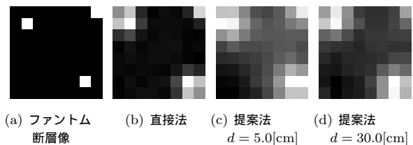
図 3 再構成結果
