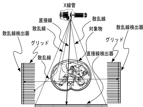
図 1 提案法体系
